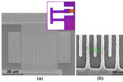
(a) Structura SAW single resonator cu 150 digiti/interdigiti având 170 nm latime; insertul prezintă întreaga structură; (b) detaliu al nanolitografiei [A. Müller, International Microwave Symposium -IMS 2014, 1-6 June, Tampa, USA pp 46-48]
