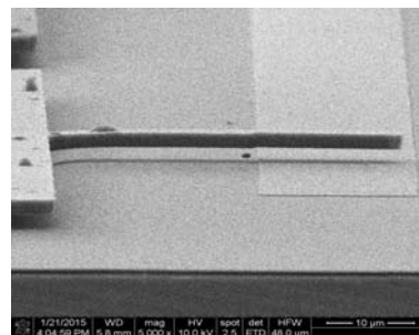
Imaginea SEM a cantileverului din polisiliciu dopat pentru masuratori vibrationale
