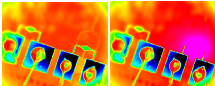
a) Hartă termică a suprafețelor microgripperului în situația inițială, fără încălzirea dispozitivului prin efect electro-termic; b) Hartă termică care surprinde încălzirea rezistenței electrice a gripperului din partea dreaptă a imaginii
