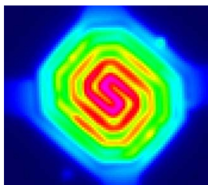
Hărți termice obținute cu microscopul în infraroșu SC 5600 + G3 L0605 / FLIR Systems .
