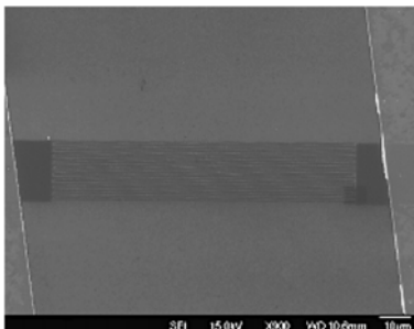
Imagine SEM a structurii, fabricate pe membrane subțiri de GaN, având digiti/interdigiti cu lățimea de 0.5 μm
